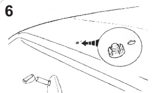
Závitořeznou část šroubku vyčnívající na základnu antény našroubovat do střešního otvoru
